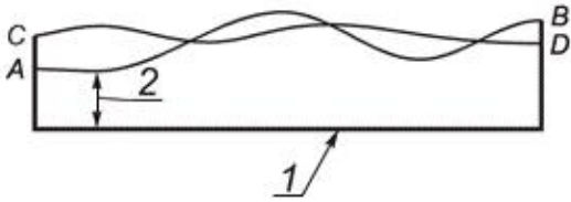
Рисунок 10.1 - Продольный профиль рельсовых ниток
