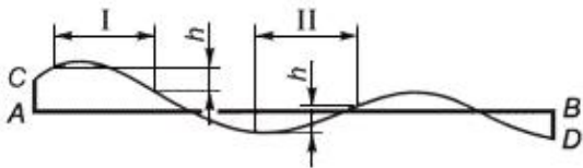
Рисунок 10.2 - Условная схема разностей отметок рельсовых ниток
