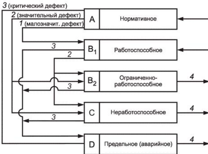
Рисунок 5.1 - Основные технические состояния (А, В(1), В(2), С, D) и изменяющие их события
